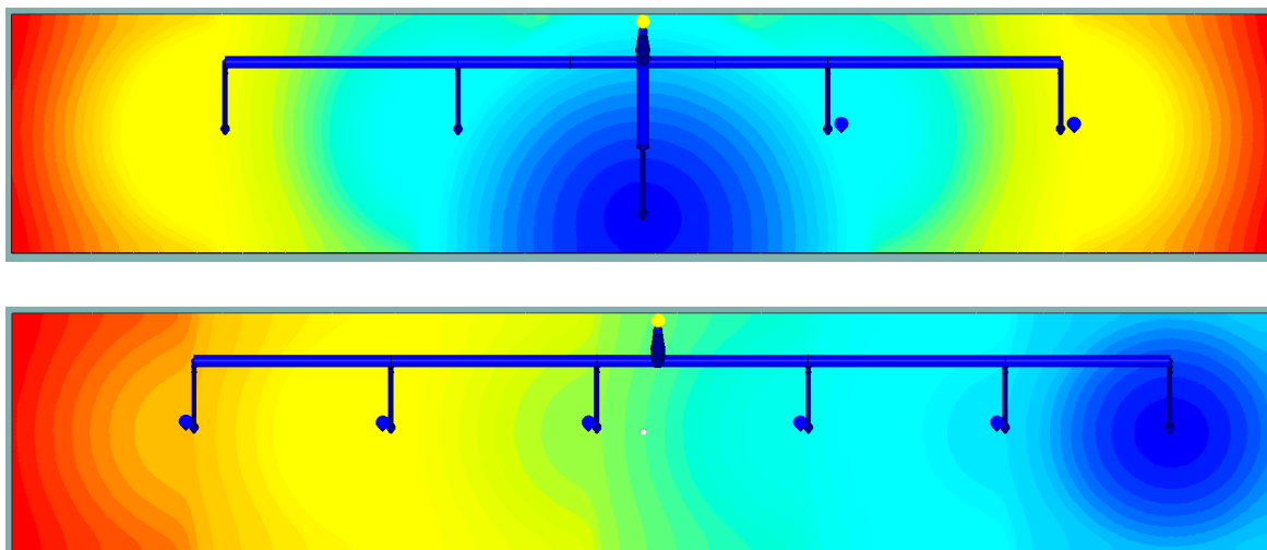
Obr. 1: Optimalizované polohy horkých trysek, výše pro systém s 5 HT, níže pro 6 HT. (Tavenina plní tvarovou dutinu postupně od míst zobrazených modře po červené oblasti.)
