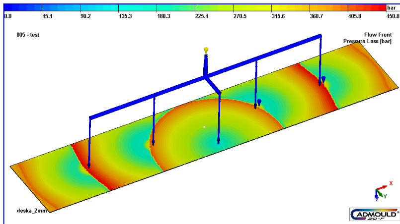
Obr. 2 a: Vstřikovací tlak pro systém s 5 horkými tryskami
