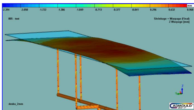
Obr. 3: Redukovaná deformace ve směru osy z, konstrukce s 5 HT a se 6 HT
