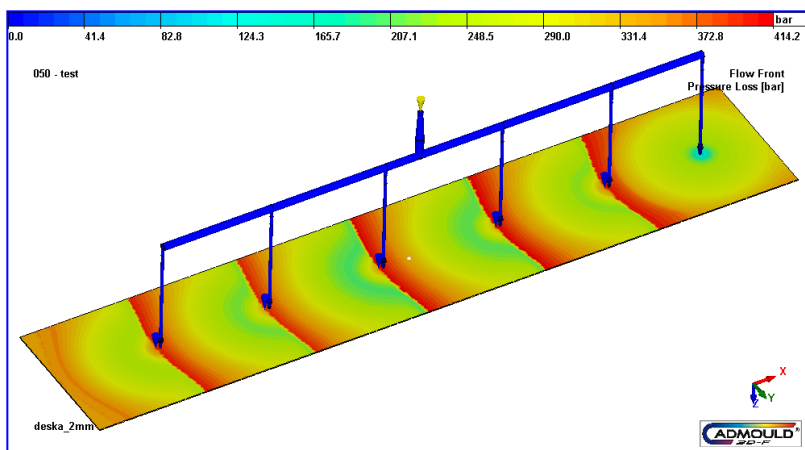
Obr. 2 b: Vstřikovací tlak pro systém se 6 horkými tryskami
