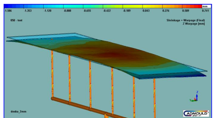
Obr. 3: Redukovaná deformace ve směru osy z, konstrukce s 5 HT a se 6 HT
